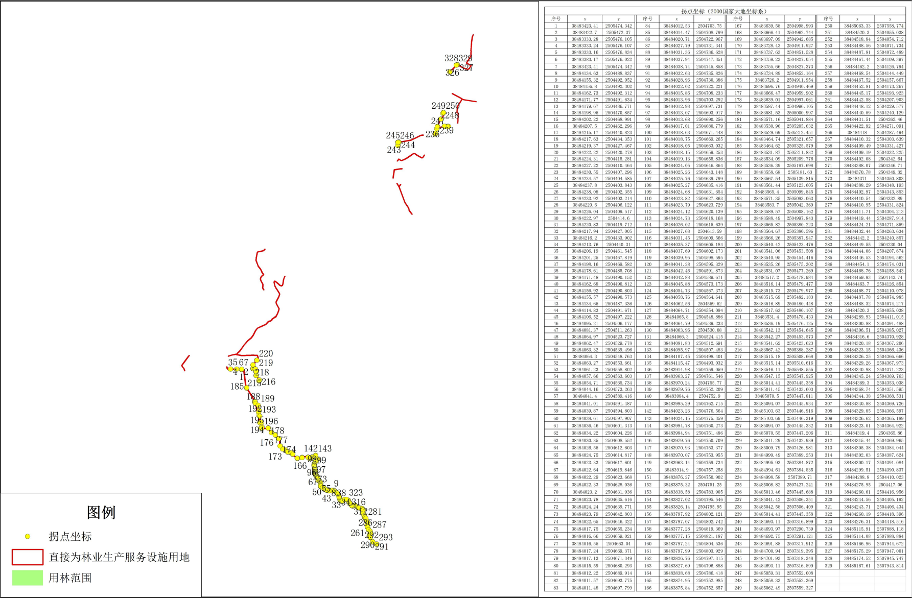
凤凰山（航城片区）山洪截滞工程地理位置示意图
