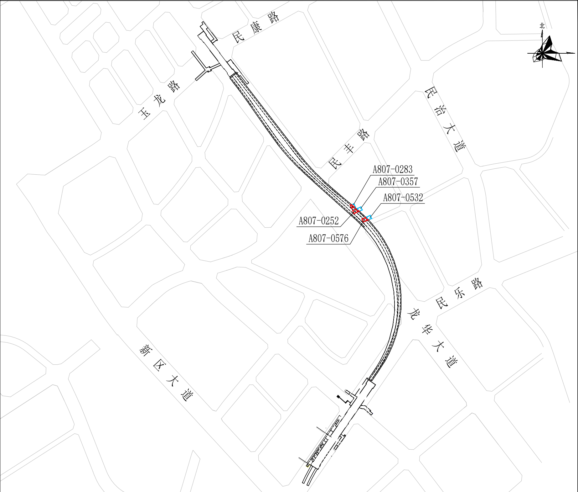
轨道交通27号线一期工程白石龙站-民康站区间与A807-0532、0576、0357、0252、0283宗地相交关系平面图
