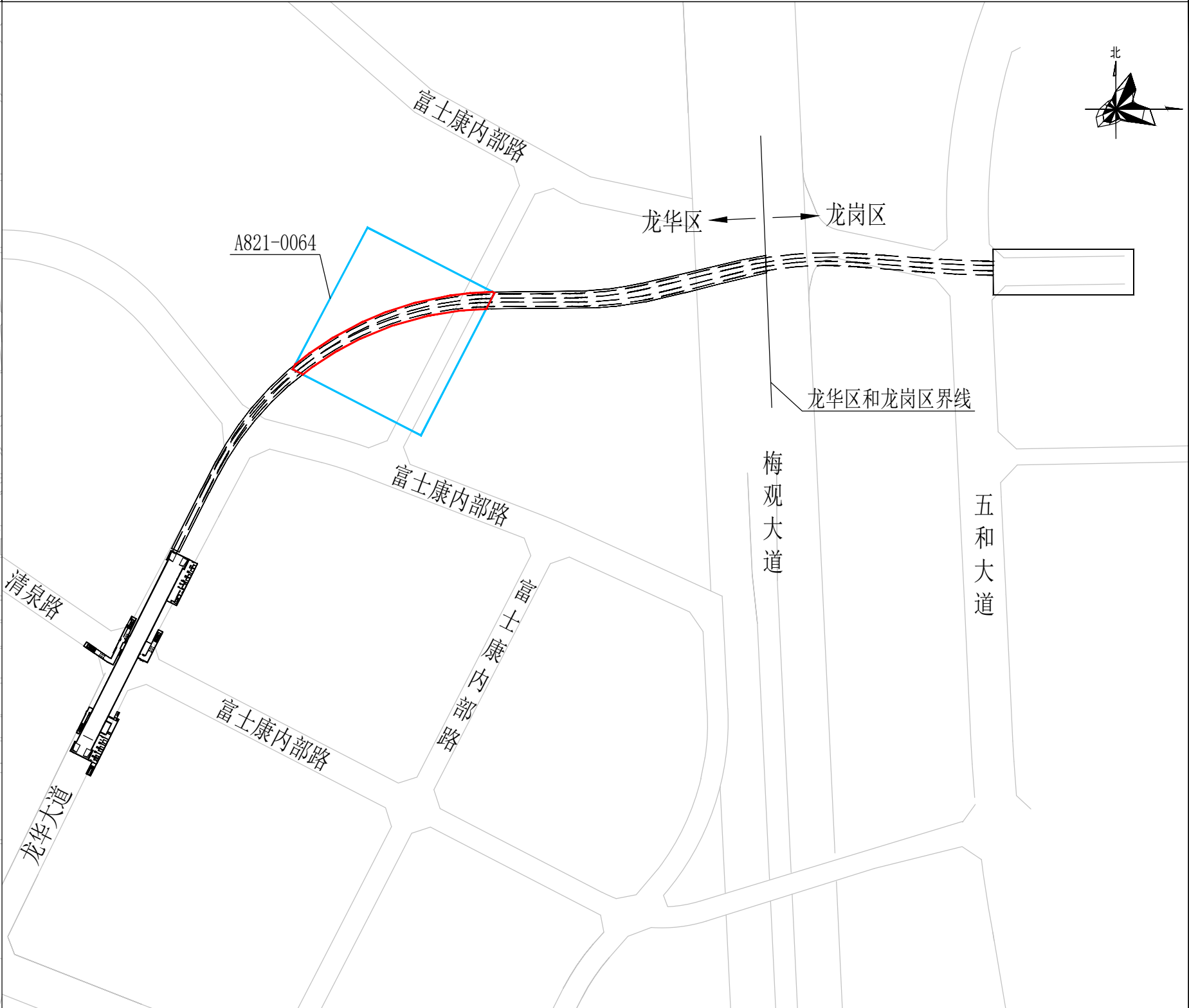
轨道交通27号线一期工程富康站-岗头西站区间与A821-0064宗地相交关系平面图
