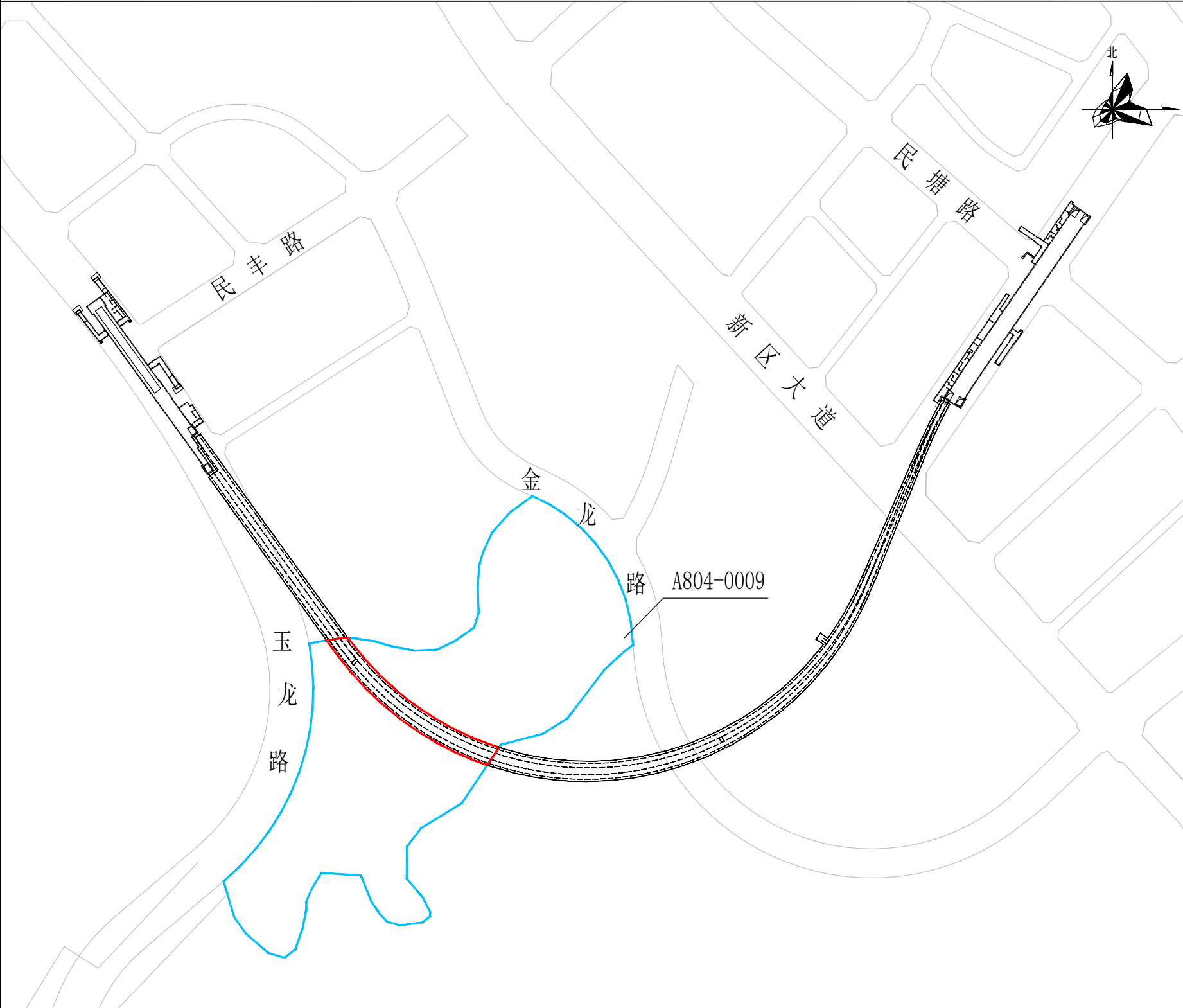
轨道交通27号线一期工程民丰路站-白石龙站区间与A804-0009宗地相交关系平面图
