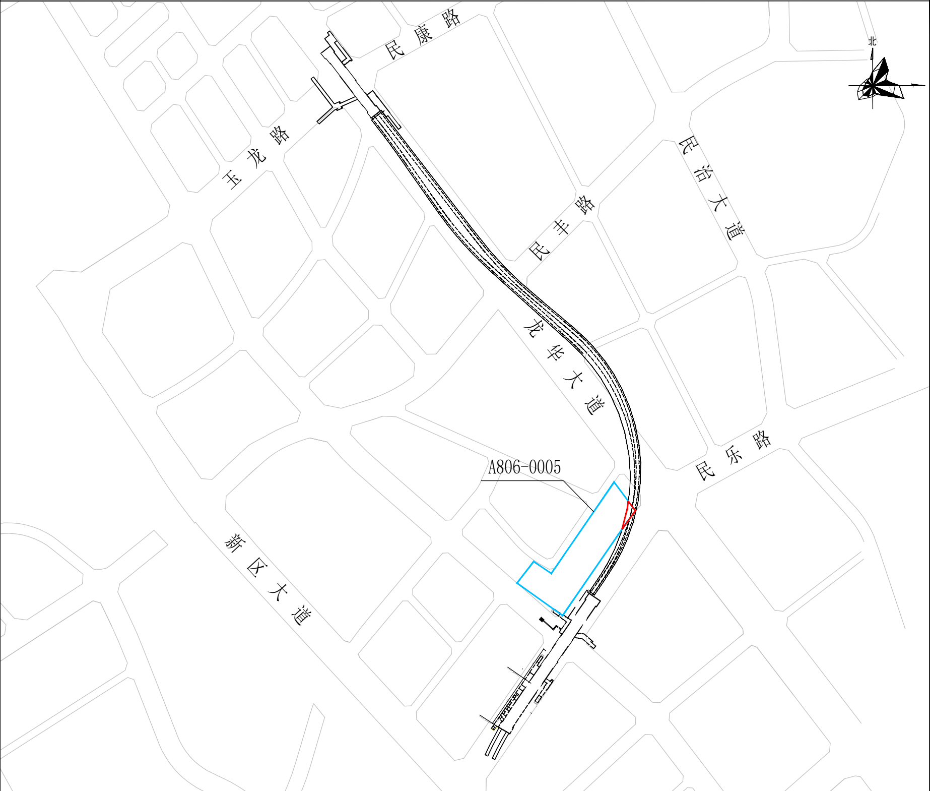
轨道交通27号线一期工程白石龙站-民康站区间与A806-0005宗地相交关系平面图
