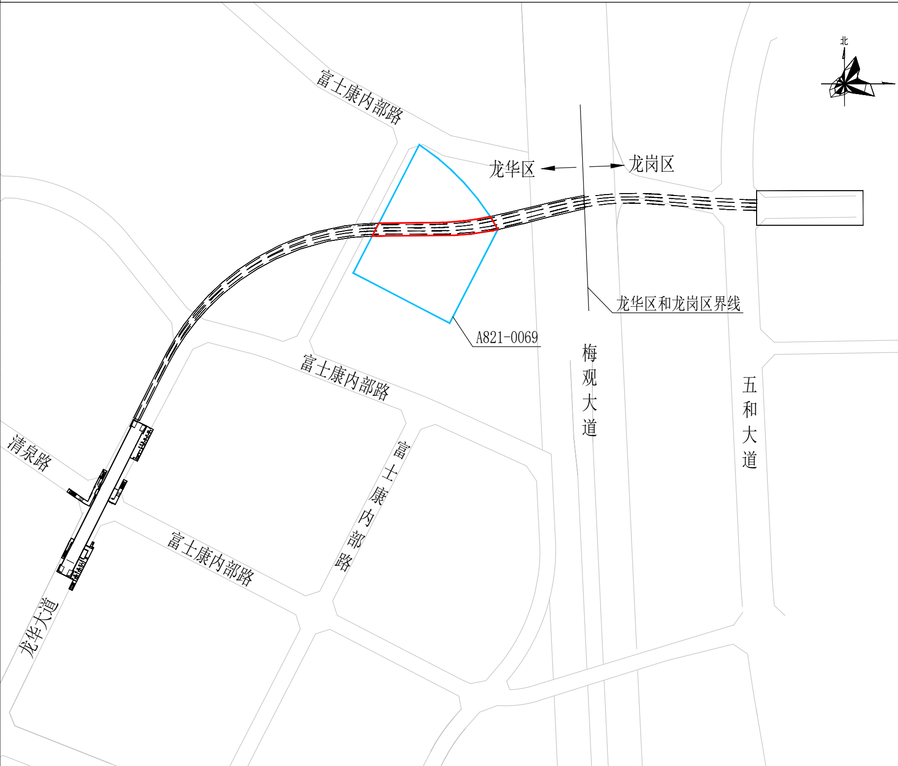
轨道交通27号线一期工程富康站-岗头西站区间与A821-0069宗地相交关系平面图
