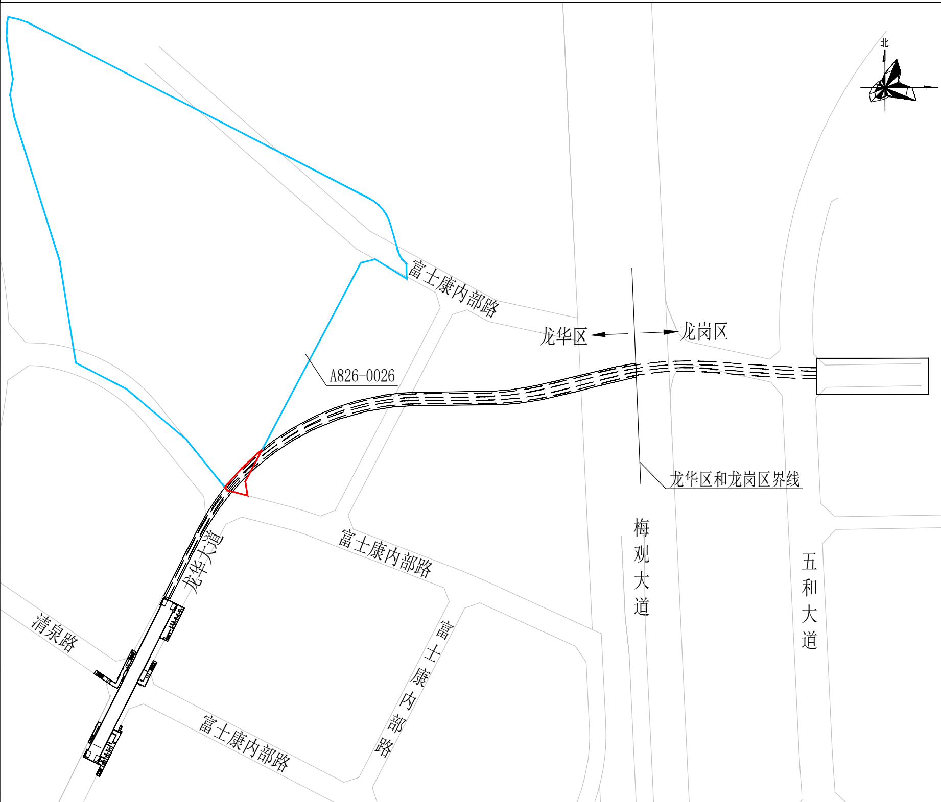
轨道交通27号线一期工程富康站-岗头西站区间与A826-0026宗地相交关系平面图
