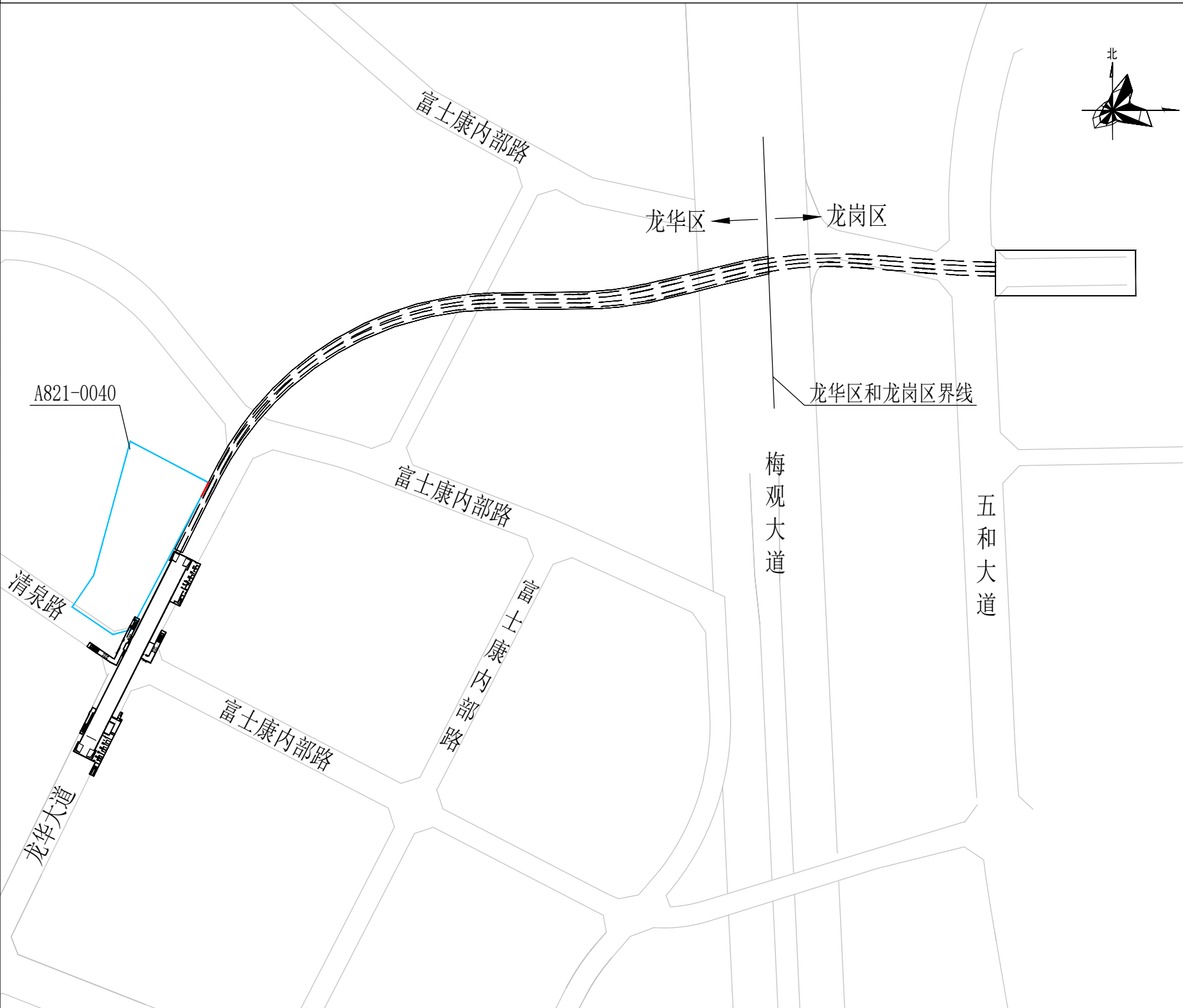
轨道交通27号线一期工程富康站-岗头西站区间与A821-0040宗地相交关系平面图
