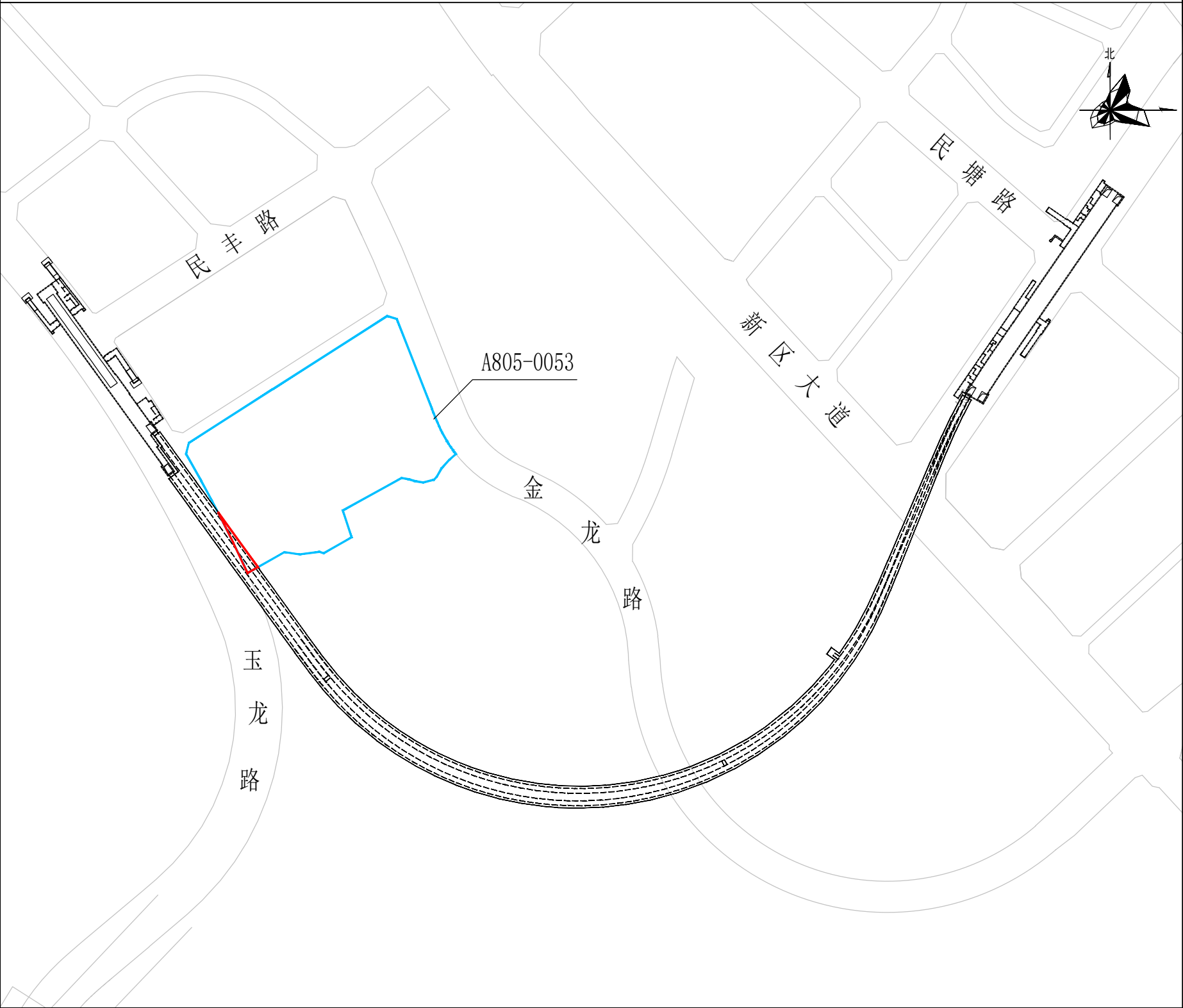
轨道交通27号线一期工程民丰路站-白石龙站区间与A805-0053宗地相交关系平面图
