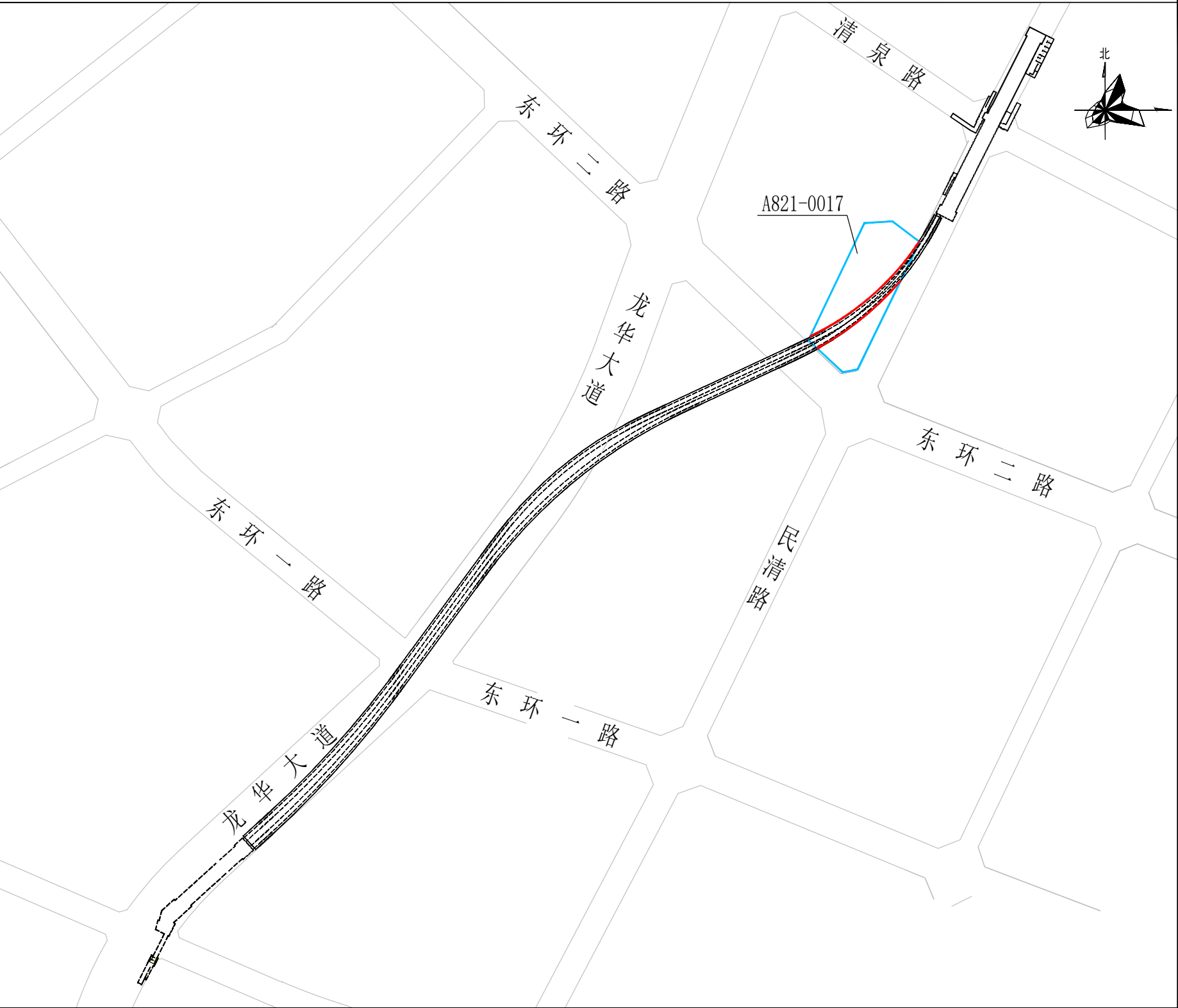
轨道交通27号线一期工程油福站-富康站区间与A821-0017宗地相交关系平面图
