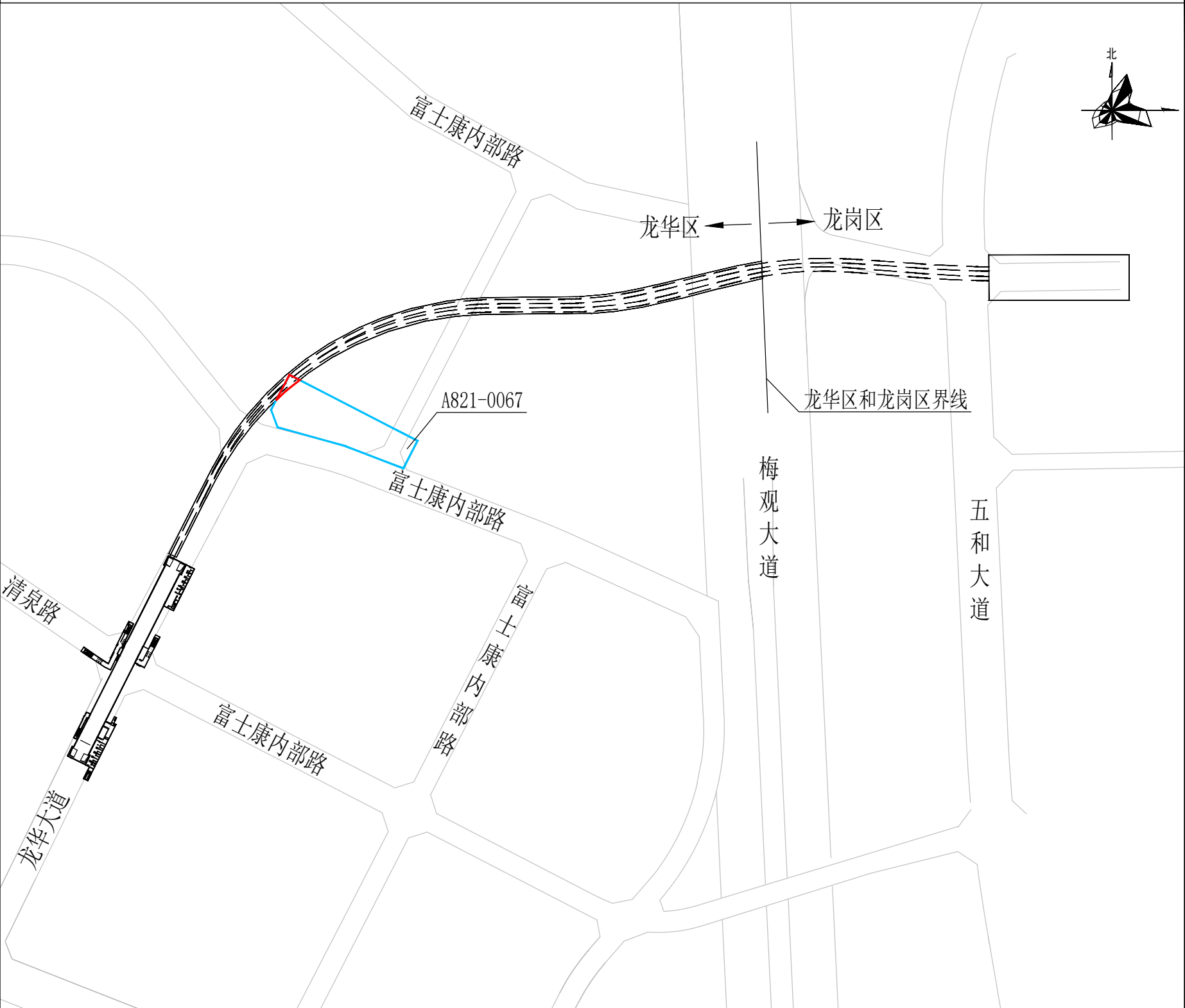
轨道交通27号线一期工程富康站-岗头西站区间与A821-0067宗地相交关系平面图
