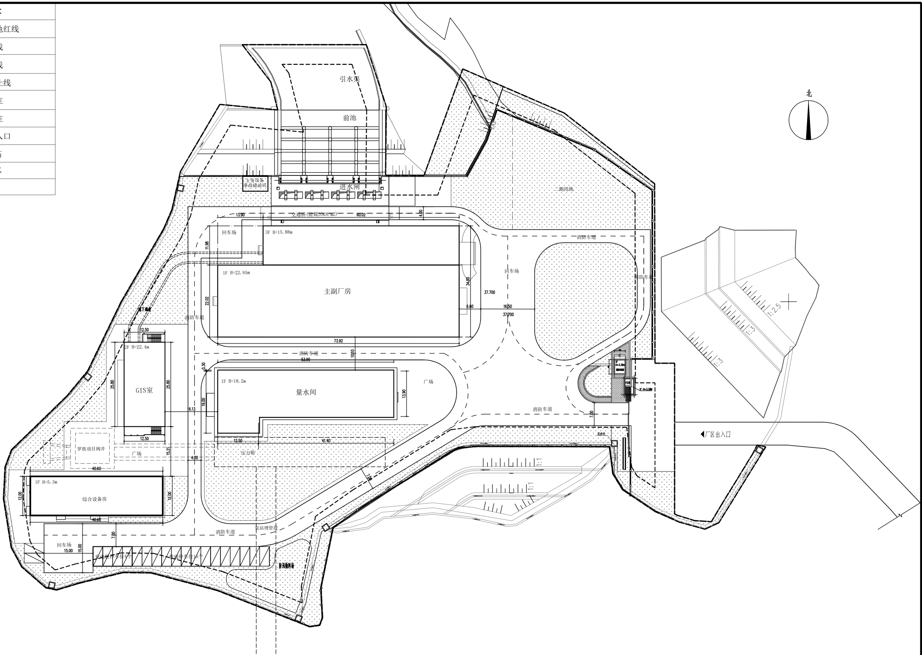
D1标罗田泵站总平面布置图 1:300
