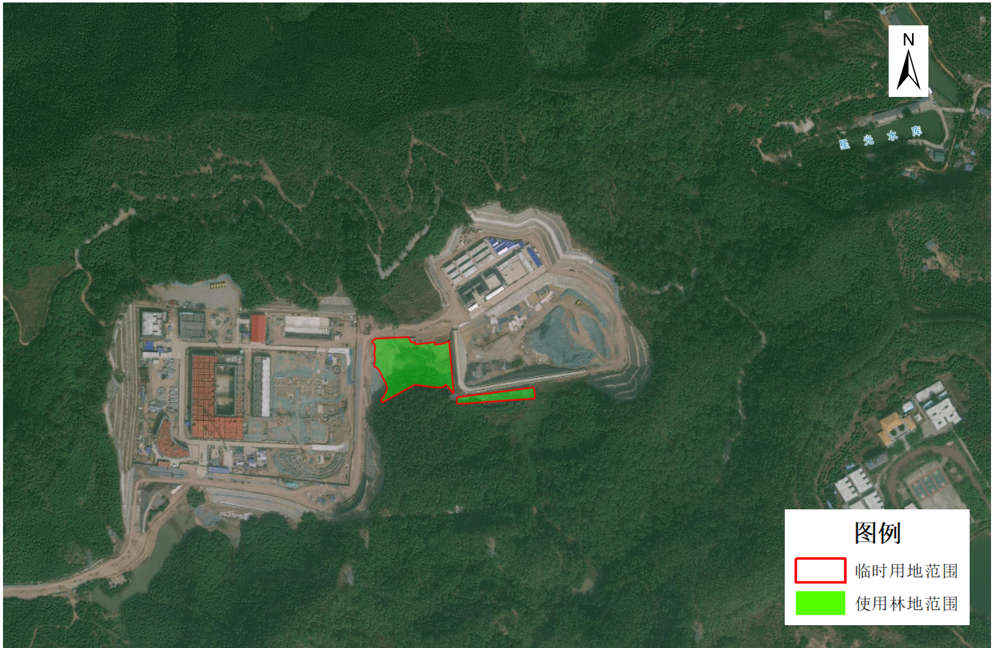
光明能源生态园填埋区边坡地理位置示意图
