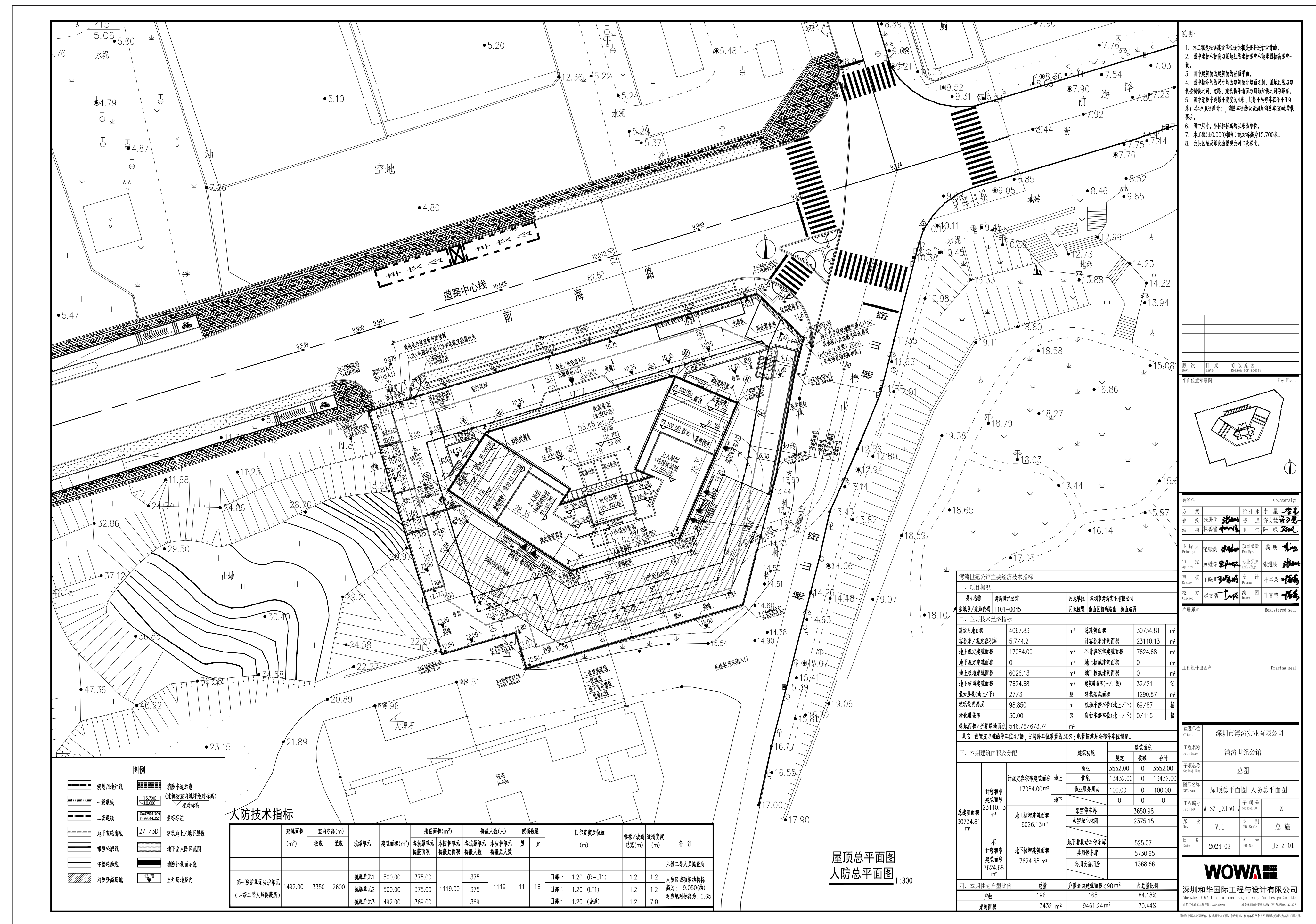
原总平面图
