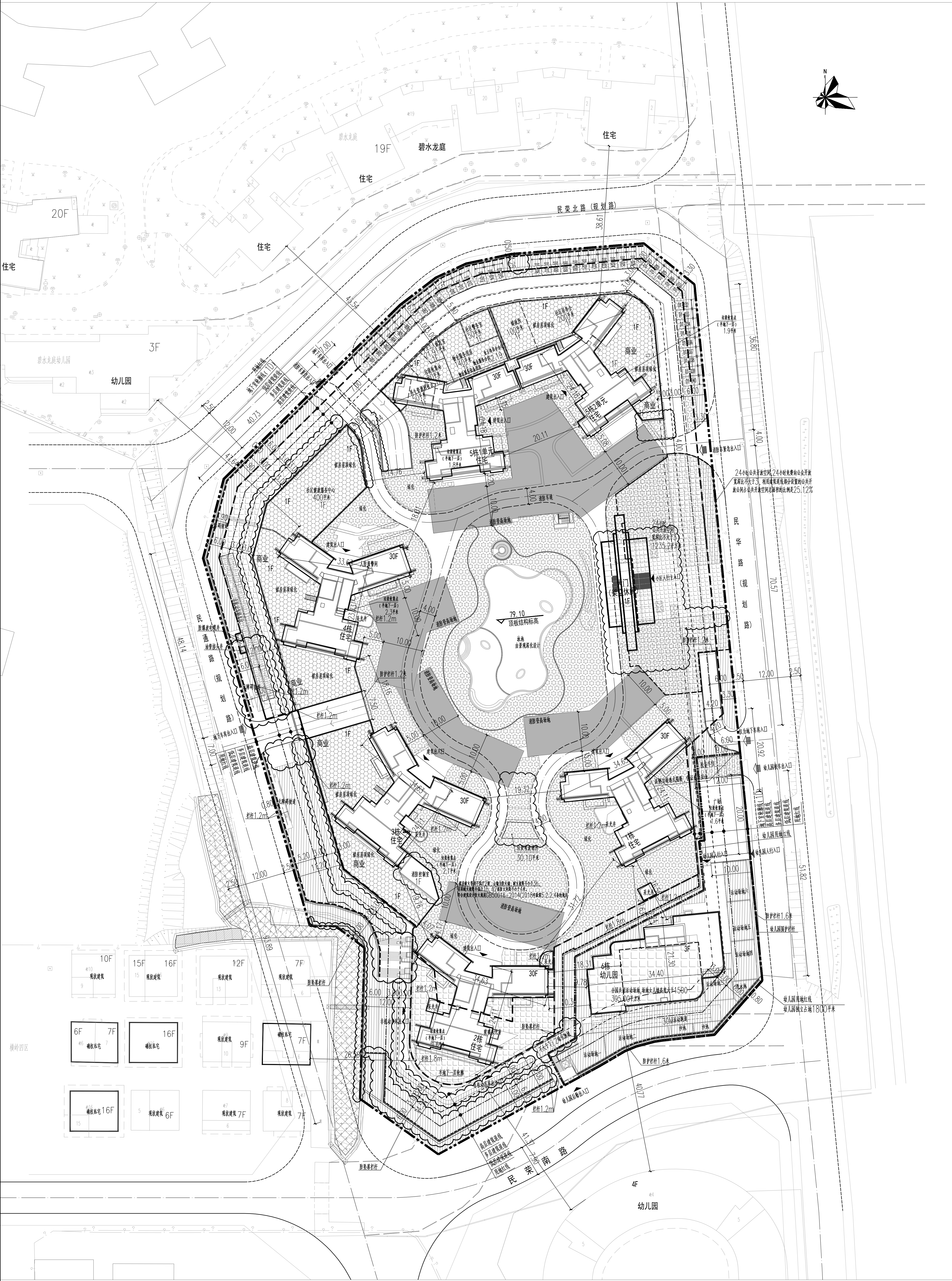
总平面图 1:400
