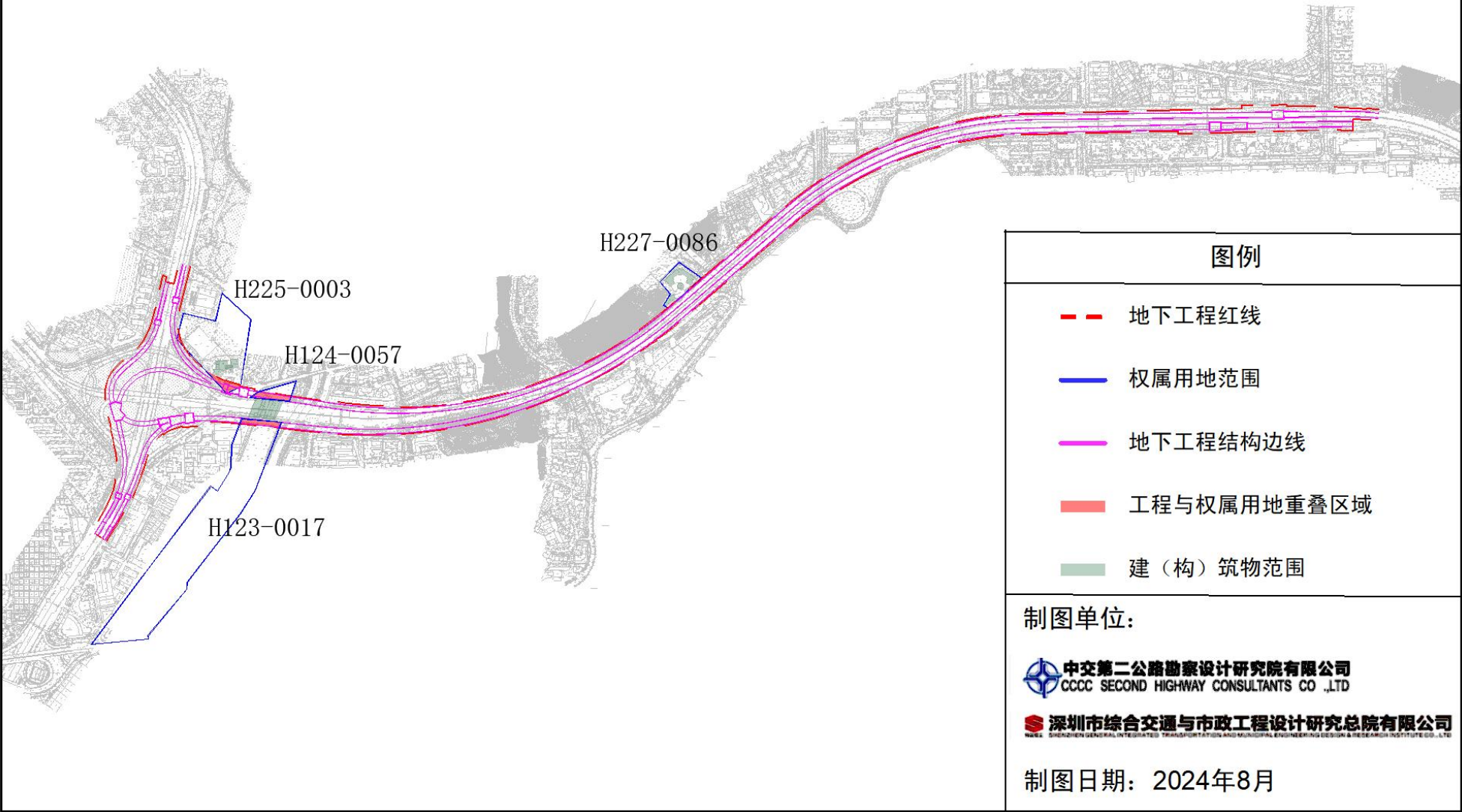
罗沙路改扩建工程（地下道路）与沿线相关权属相交关系总览图
