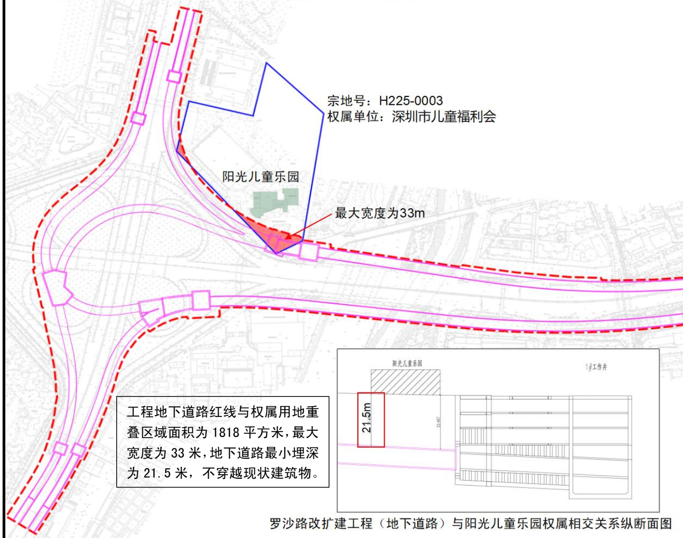
罗沙路改扩建工程（地下道路）与阳光儿童乐园权属相交关系平面图
