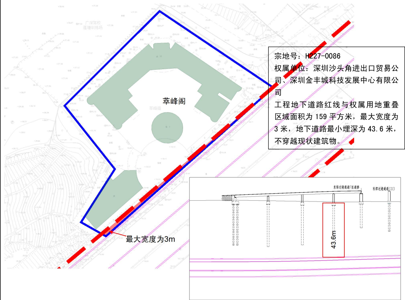
罗沙路改扩建工程（地下道路）与萃峰阁权属相交关系纵断面图
