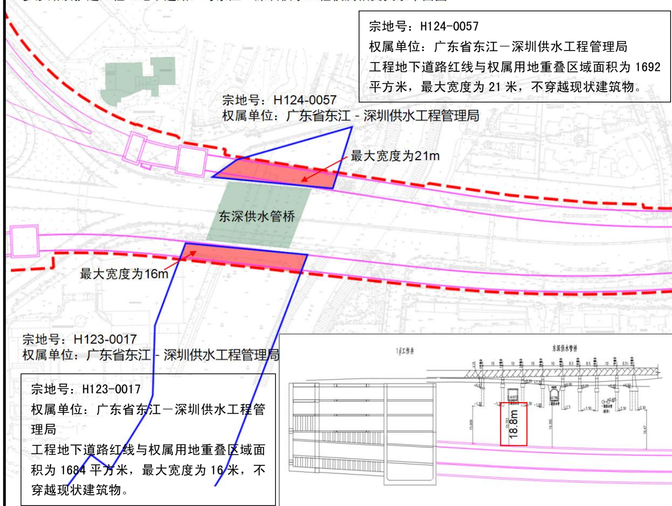
罗沙路改扩建工程（地下道路）与东江—深圳供水工程权属相交关系纵断面图
