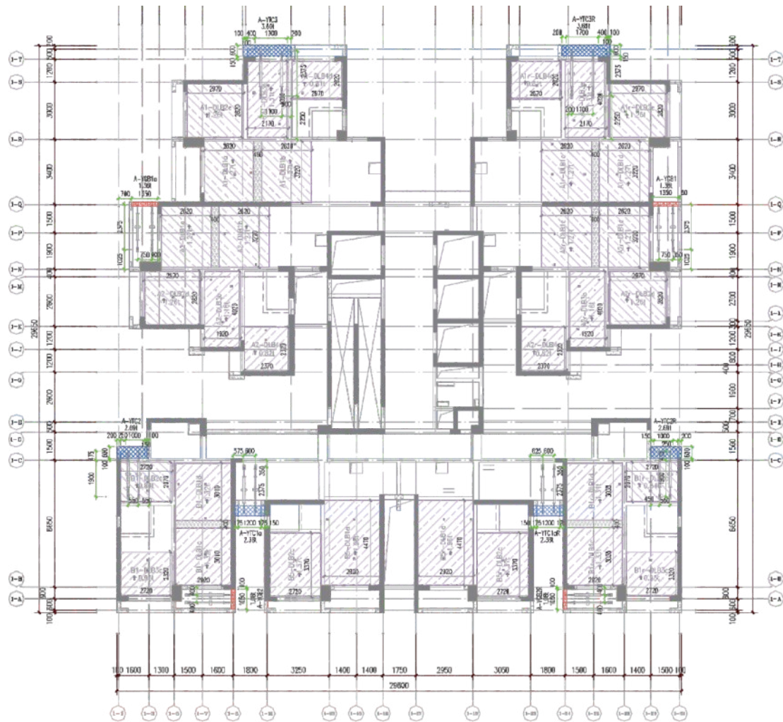
1 栋一单元预制构件平面布置图
