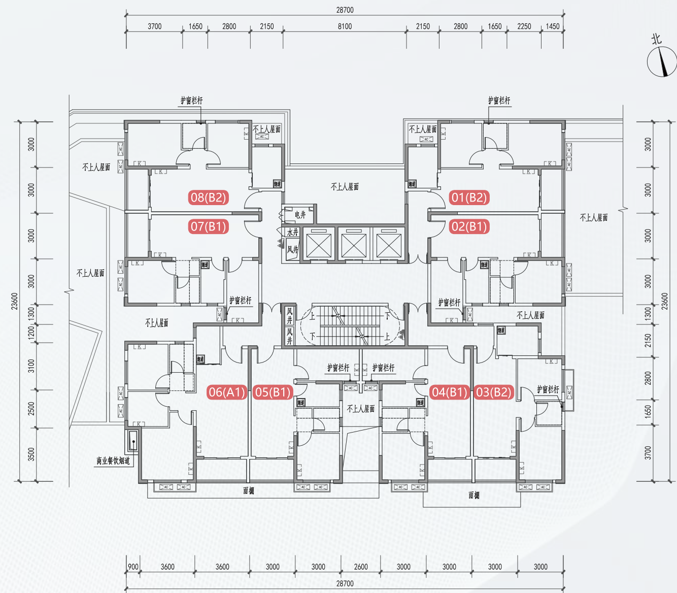
非标准层（2栋一单元2层）
