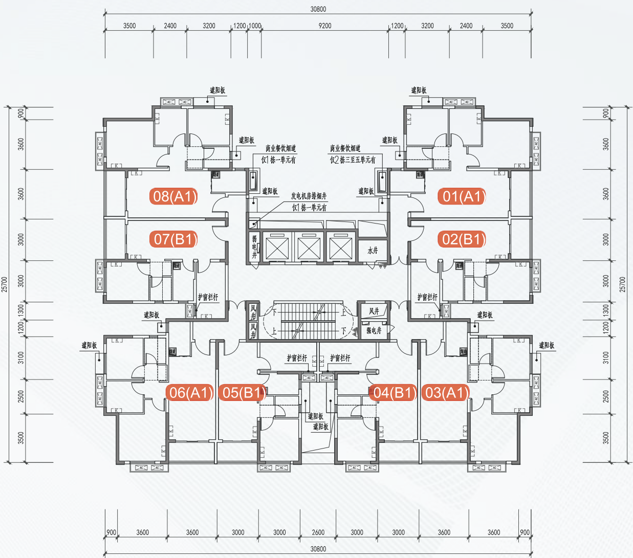
标准层（1栋一单元 3~34层、2栋三至五单元 3~33层）
