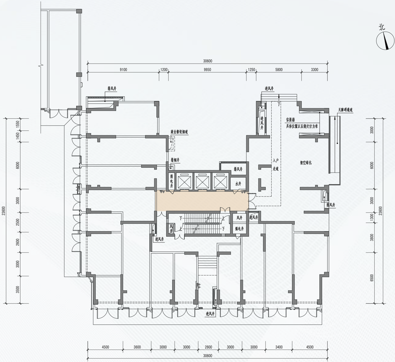
非标准层（1栋一单元1层）
