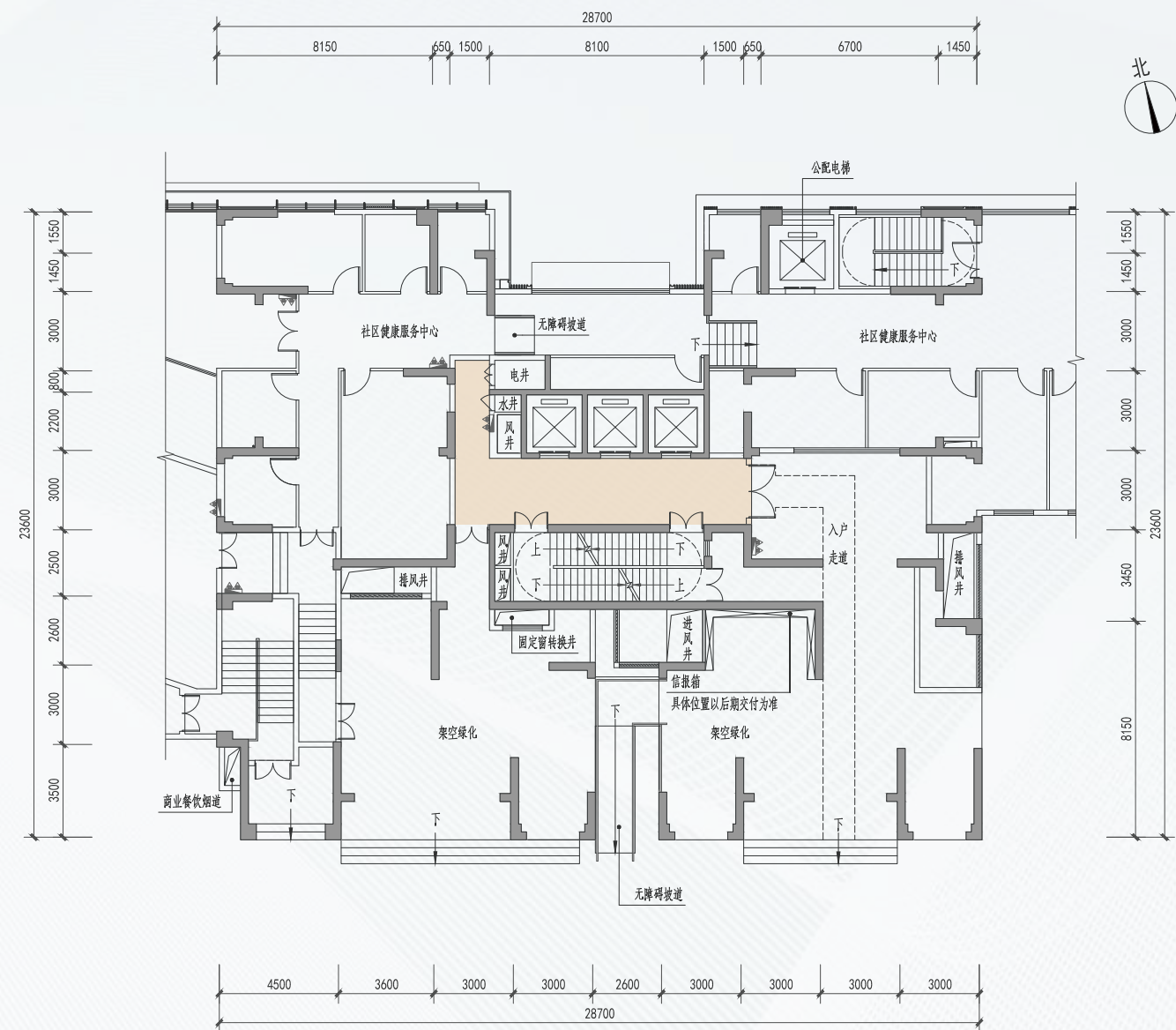
非标准层（2栋一单元1层）
