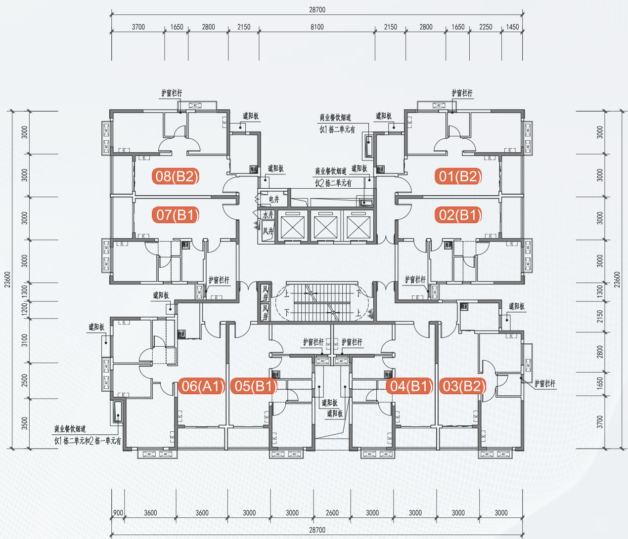
标准层（1栋二单元 3~34层、2栋一至二单元 3~33层）
