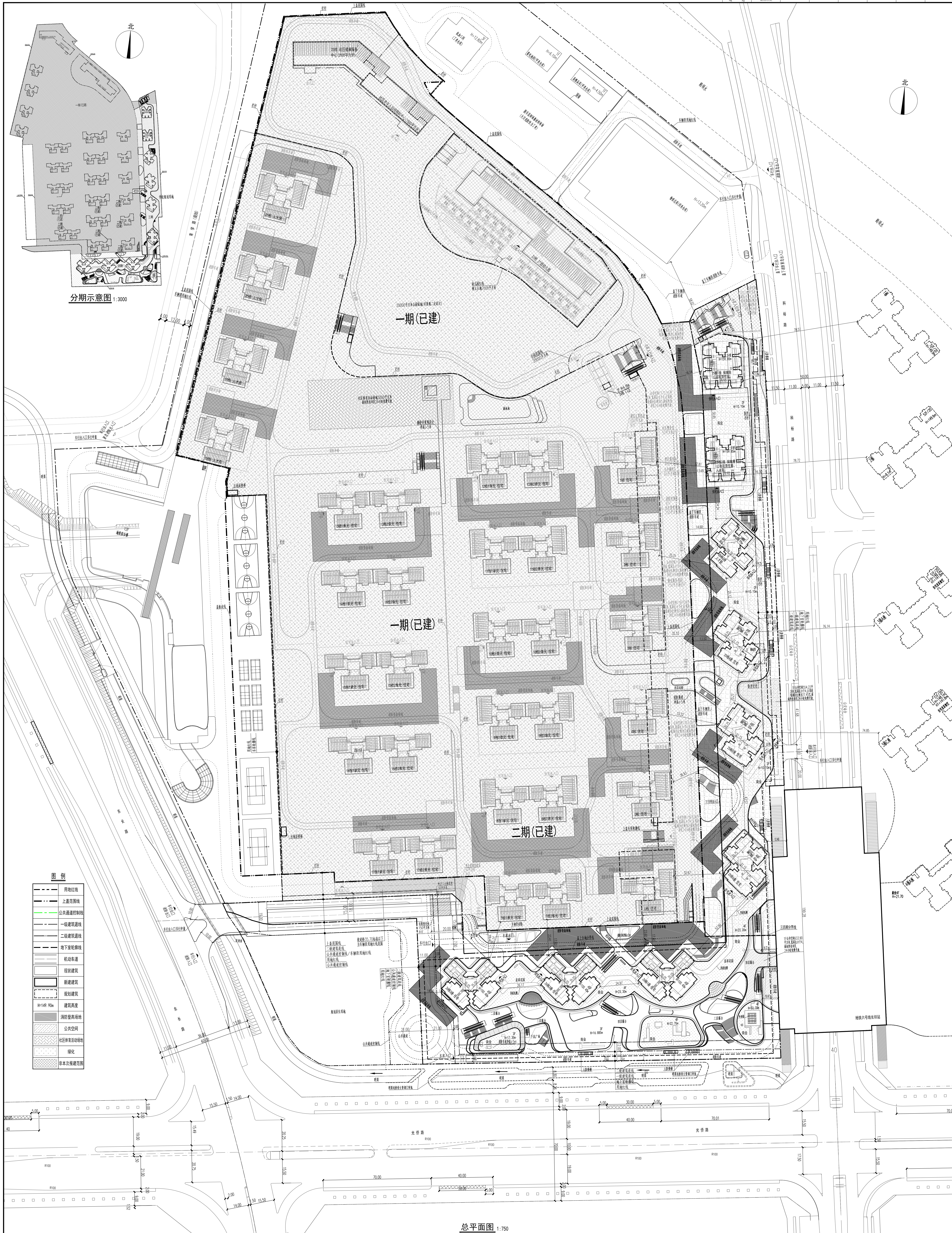
总平面图 1:750
