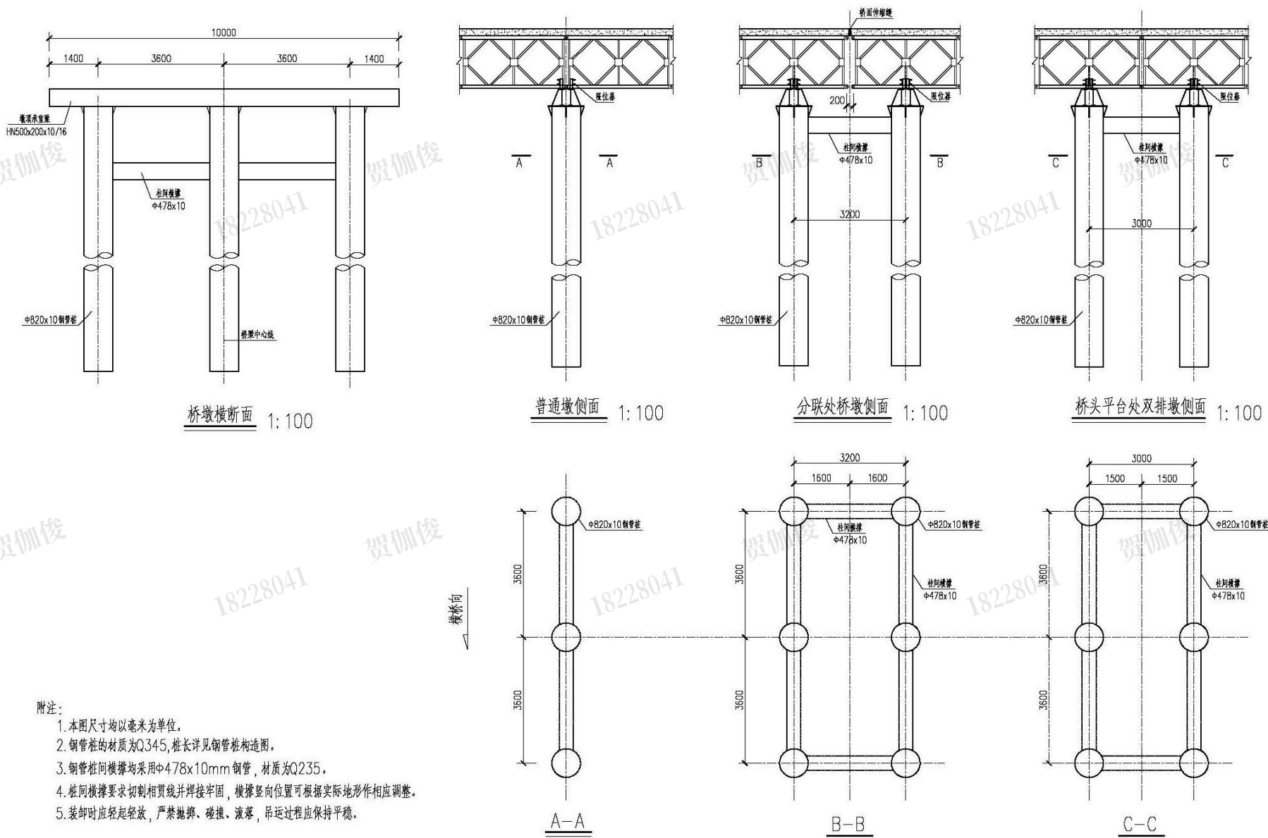
图 2.2-6 桥墩一般构造图
