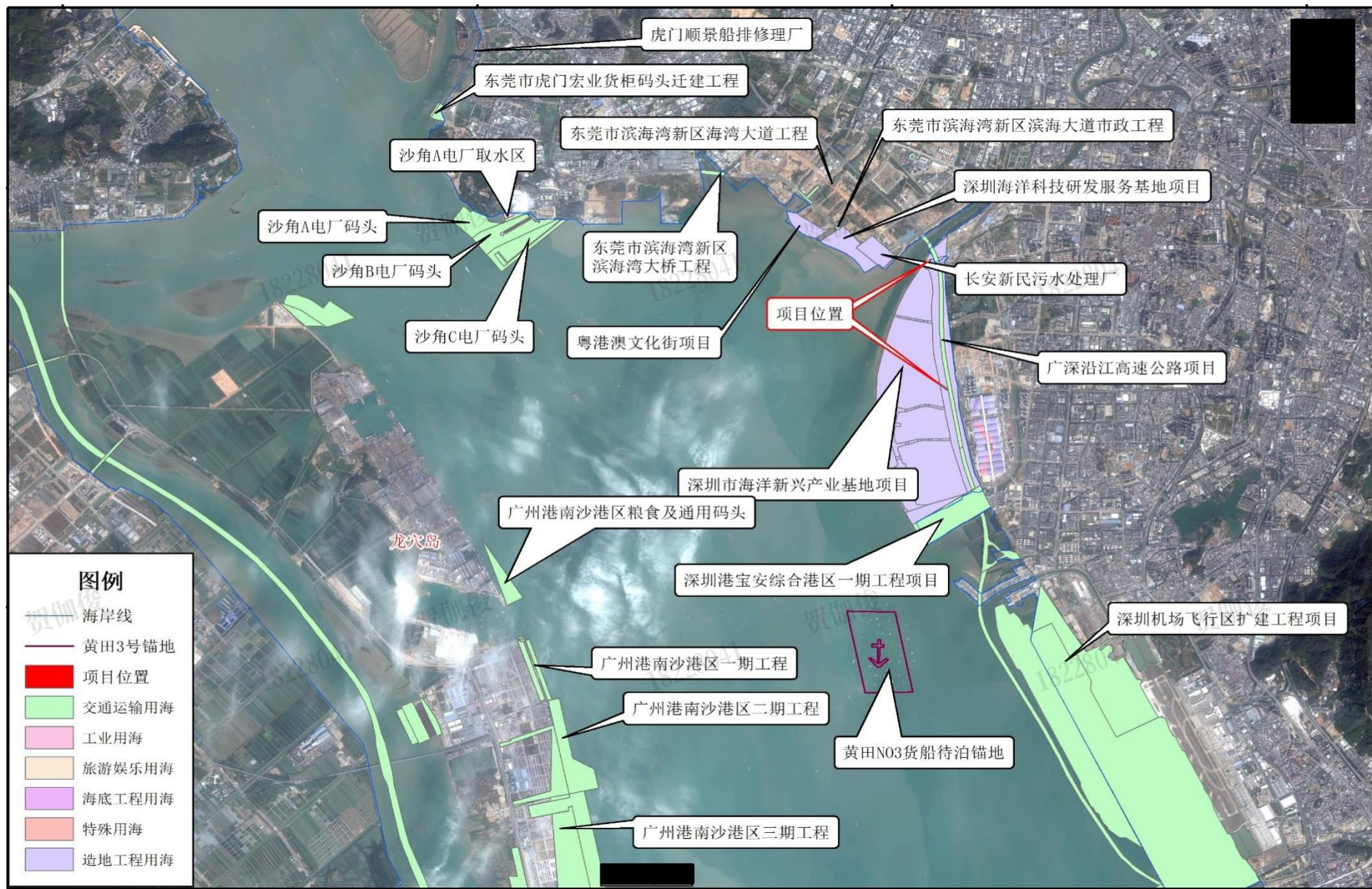
图 3.4-1 项目周边海域开发利用活动
